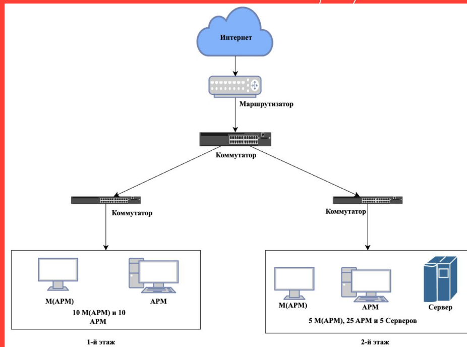
Комплекс технических средств организации
